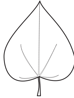
Palmate
